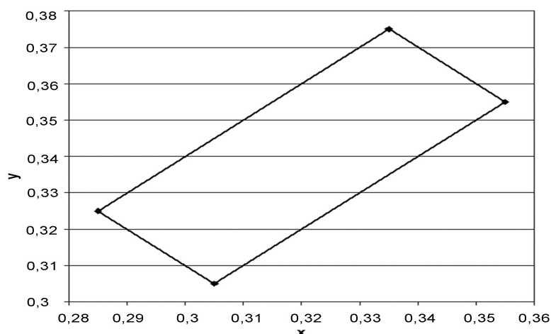
Rys. 1. Współrzędne chromatyczności x,y dla barwy białej oznakowania
