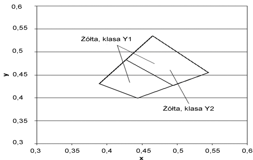
kys.2. współrzędne chromatyczne x,y dla barwy żółtej oznakowania
